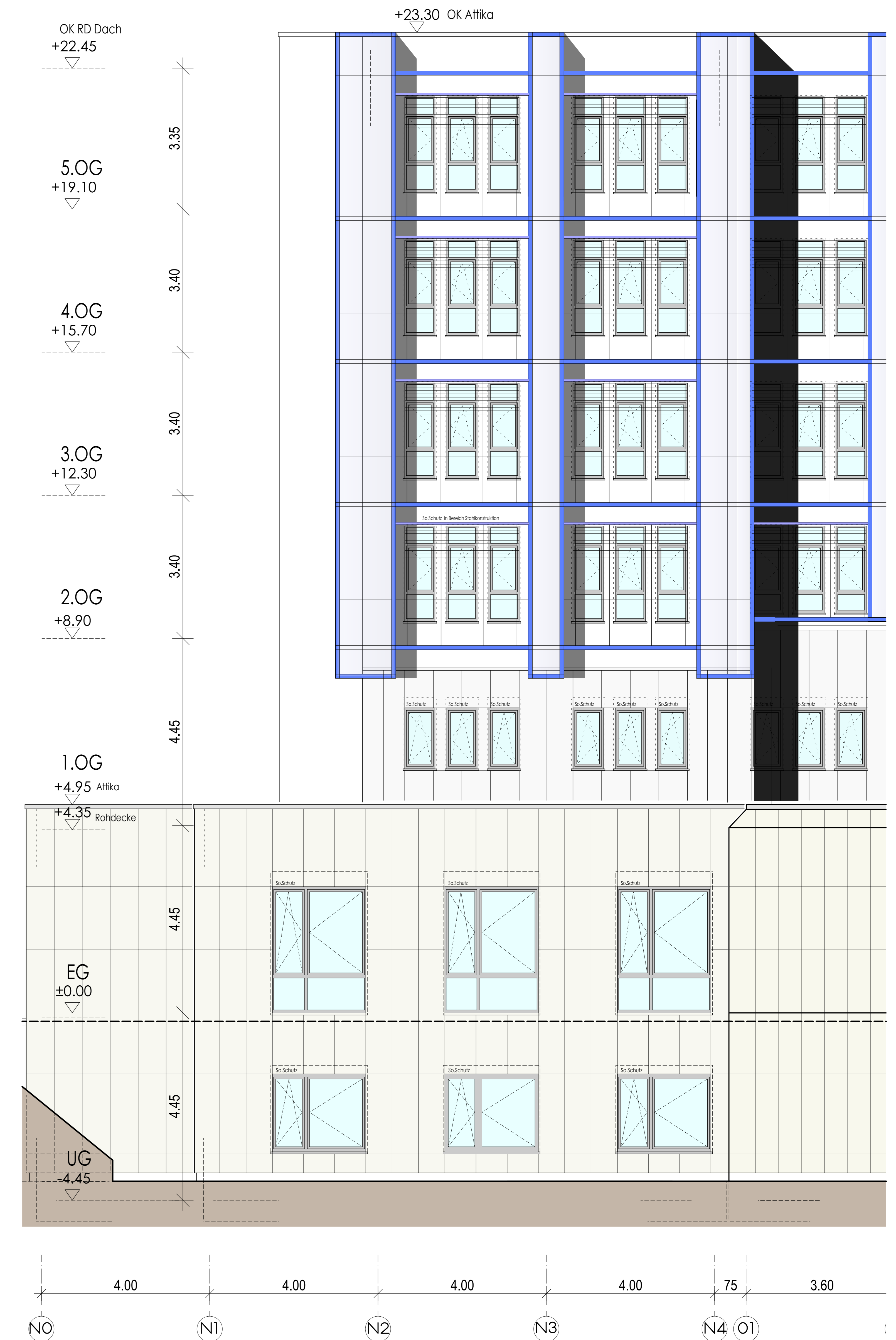
Ausschnitt Ansicht Süd
